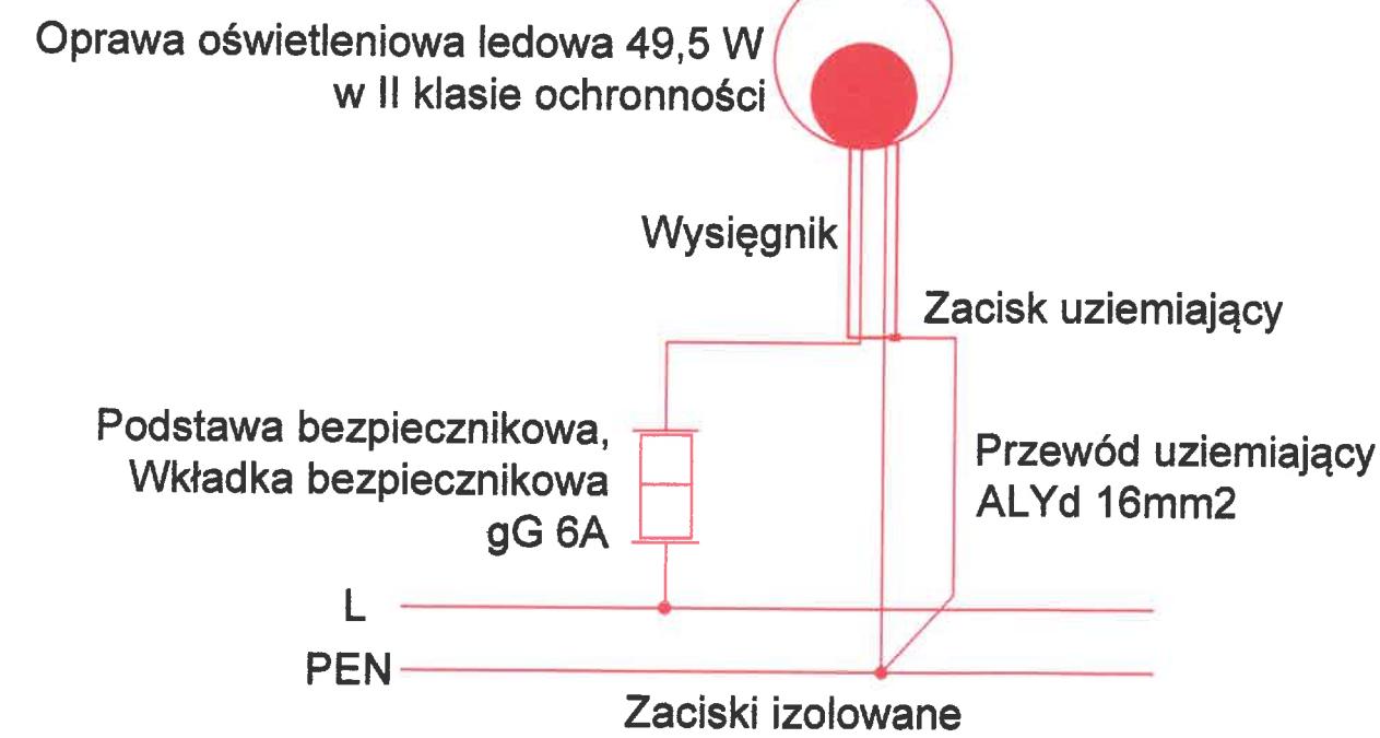
Schemat podłączenia oprawy oświetleniowej Układ sieci TN-C
